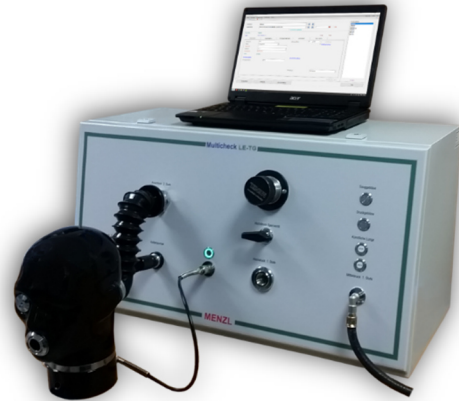
MC LE-TG mit Sonderausstattung Druckminderer Prüfkopf und Notebook
